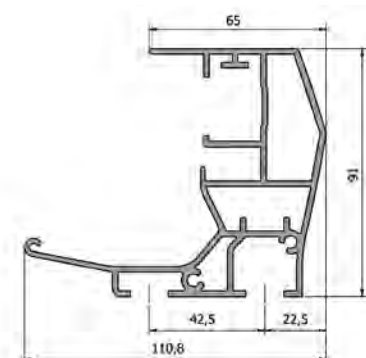
Einzelführungsschiene
