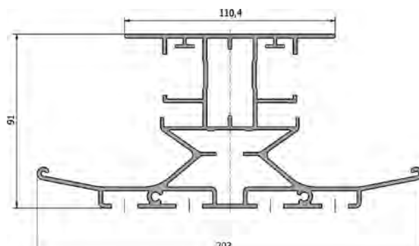
Mittenführungsschiene
