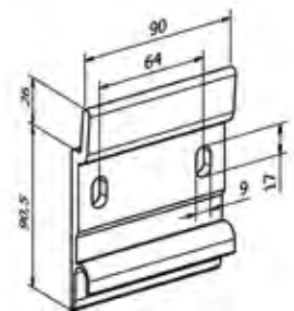
Wandkonsole bemaßt
