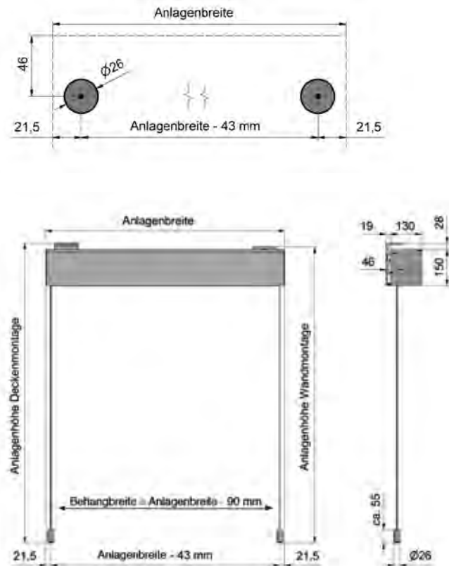
Seilabspannung Bodenmontage
