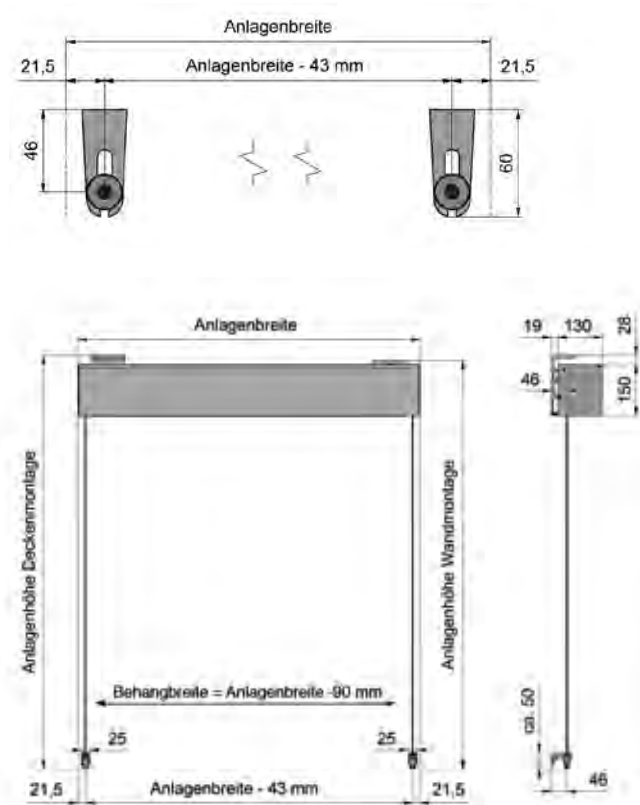
Seilabspannung gefedert
