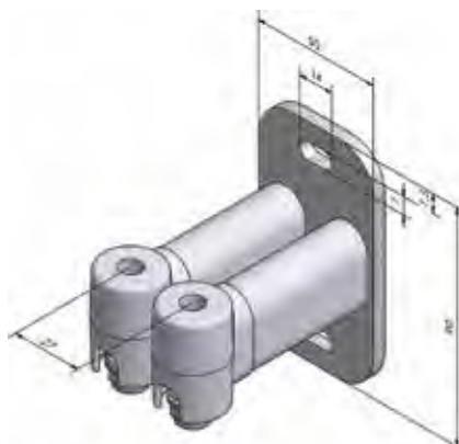
Doppelseilhalter 85 mm
