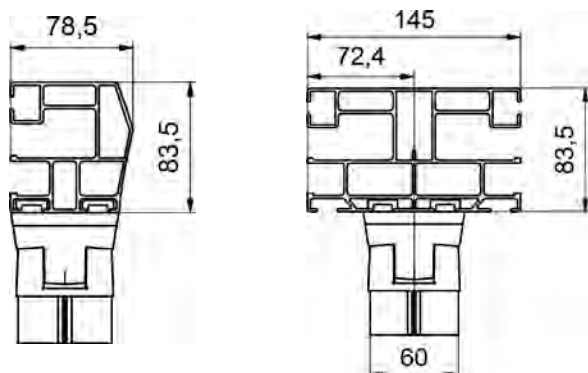
Einzelführungsschiene Mittenführungsschiene
